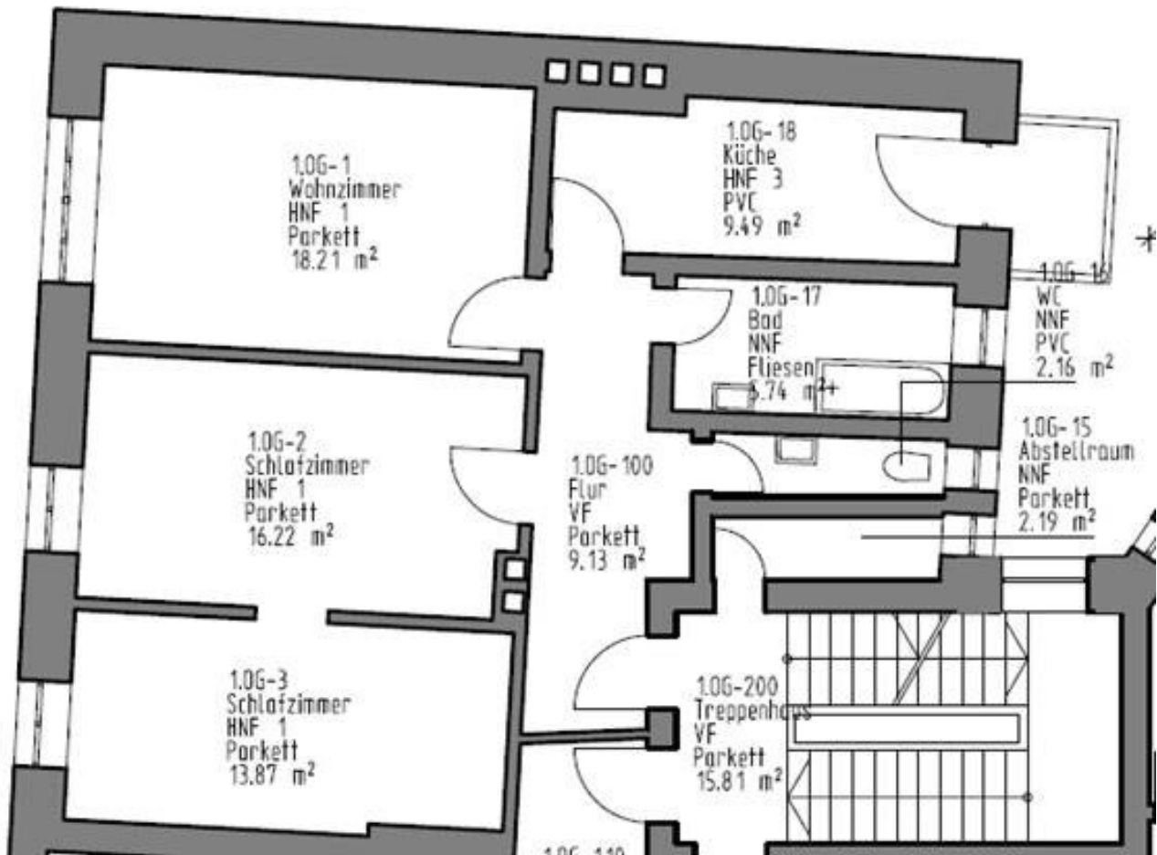
Grundriss
