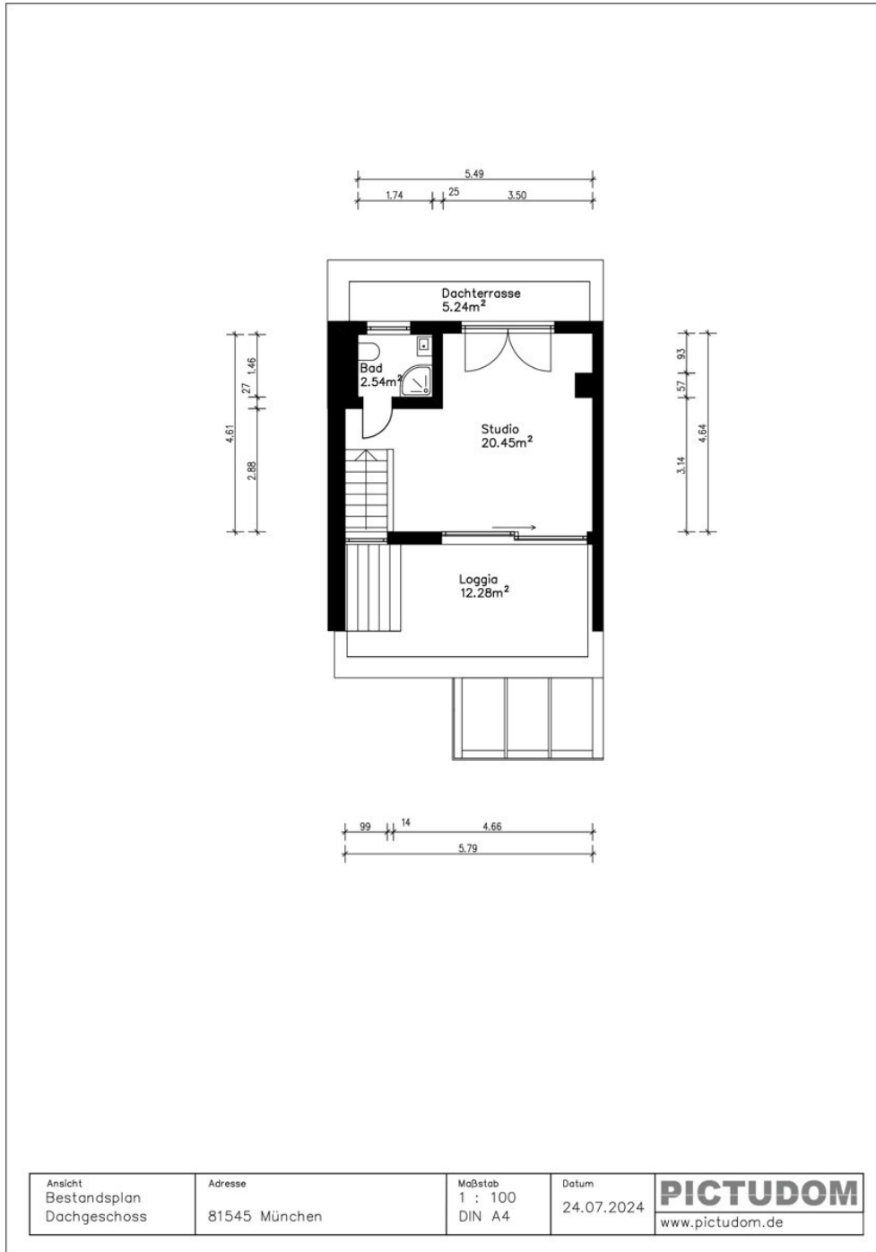
Grundriss DG_2
