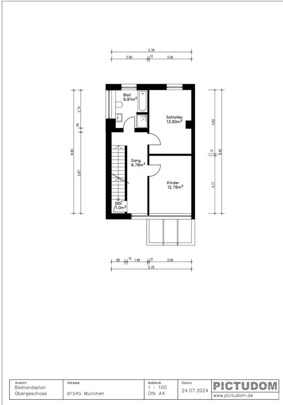
Grundriss OG
